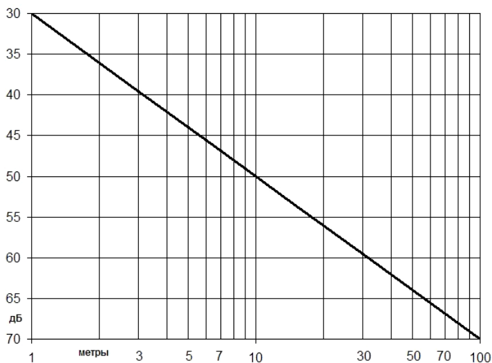
Рисунок 8. Зависимость затухания на частоте 900 МГц при горизонтальном разноразе дипольных антенн.
